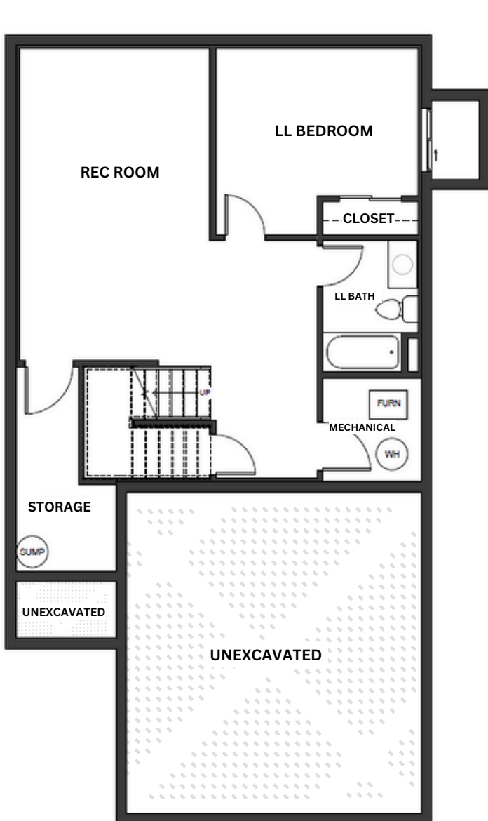
MAGNOLIA Optional Lower Level Aprx: 653 SQFT
