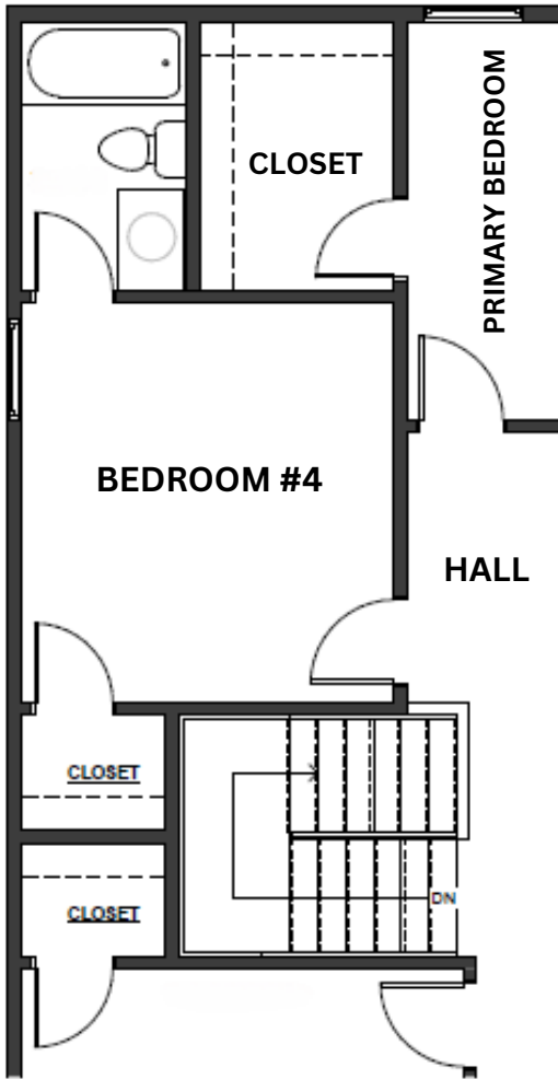
Optional 3.5-Bath Layout
